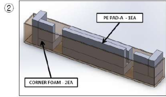
② 2. BOTTOM BOX 안에 CORNER FOAM 과 PE PAD-A를 넣는다.
