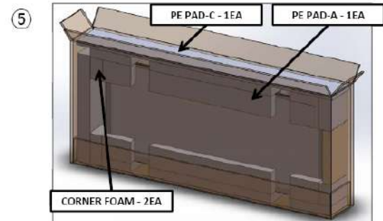
⑤ 5. CONRER FOAM과 PE PAD-A,C를 넣는다.
