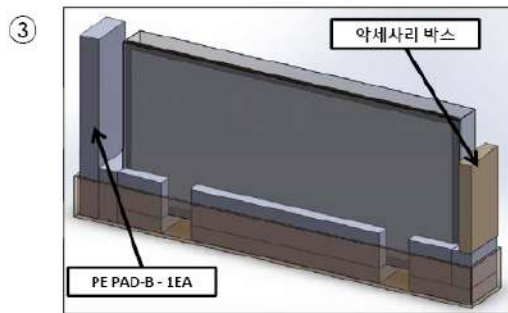
③ 3. NEP SET를 넣고, 측면에 약세사리 박스와 PE PAD-B를 넣는다.
